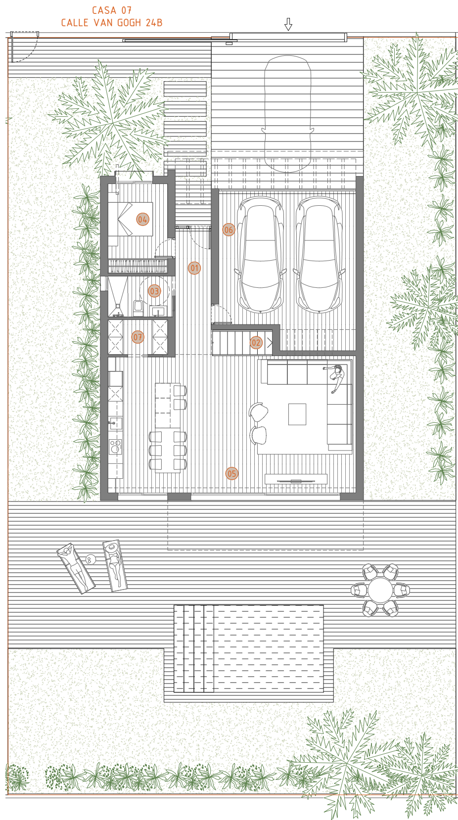
PARCELAS 7: PLANTA BAJA
