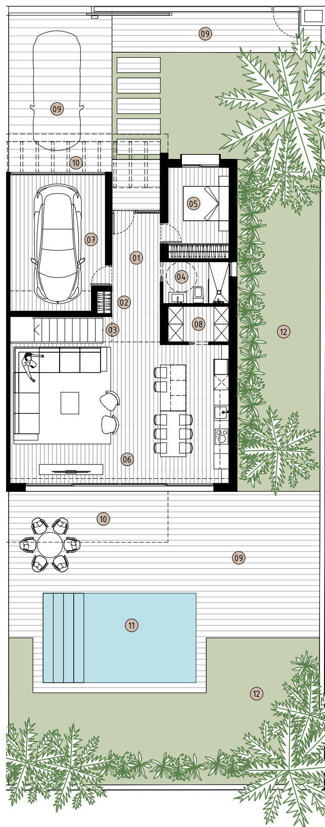
PARCELAS 7: PLANTA BAJA
