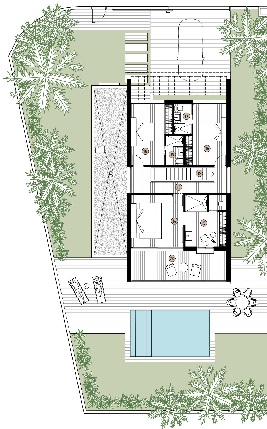
PARCELA 1: PLANTA PRIMERA
